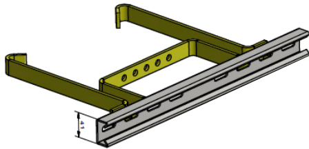
Monostrut skinne
